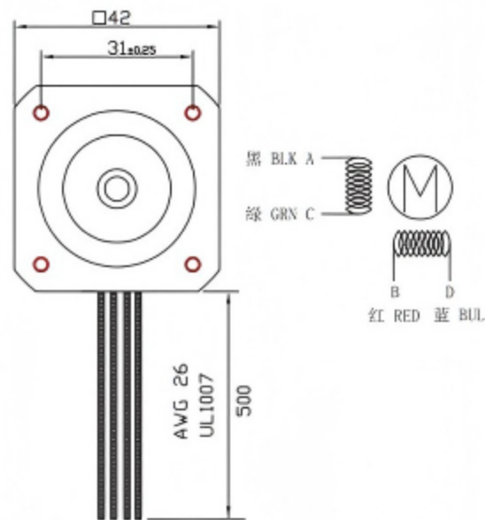
绕线图 Wiring Diagram
