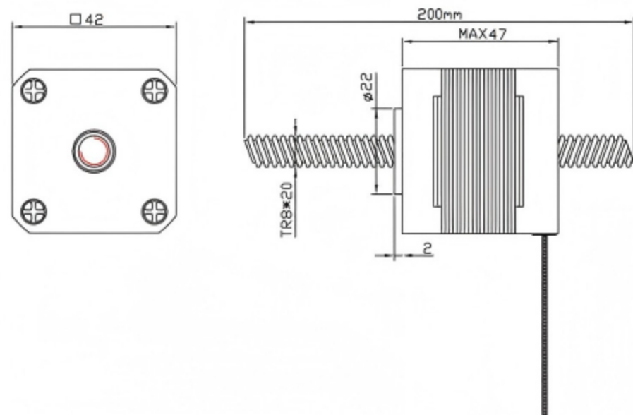
技术参数 Technique Parameter
