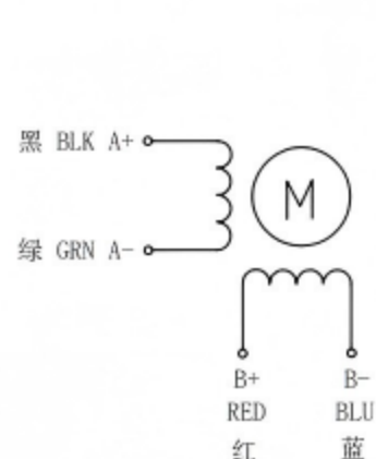
绕线图 Wiring Diagram
