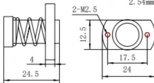
螺母尺寸图 POM材质消除
