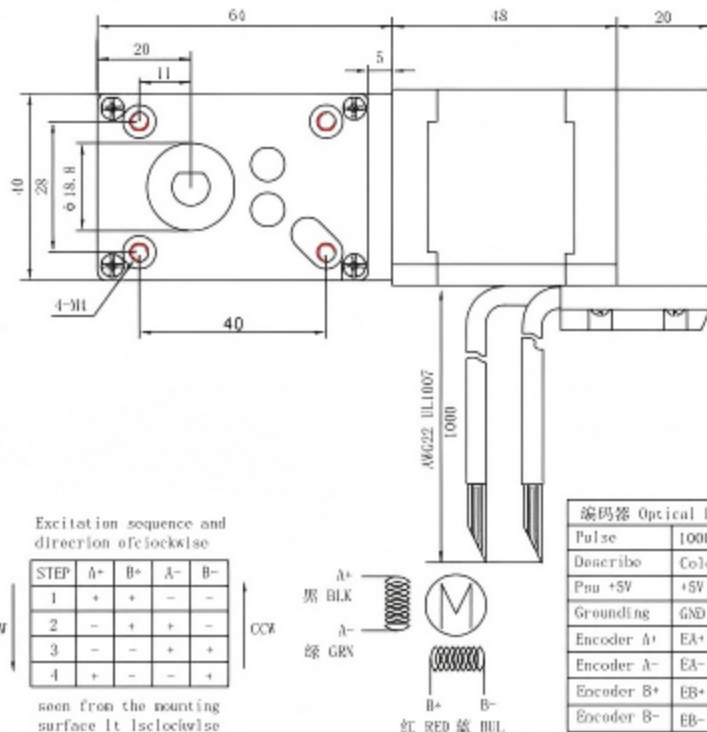
绕线图 Wiring Diagram
