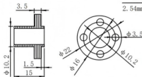
螺母尺寸图 铜材质
