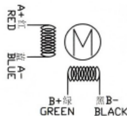
绕线图 Wiring Diagram
